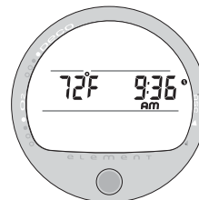
Рис. 29 Бездекомпрессионное погружение. Дополнительный экран 1
