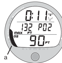
Рис. 25. Уровень насыщения кислородом
