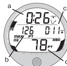
Рис. 28 Бездекомпрессионное погружение. Основной экран
