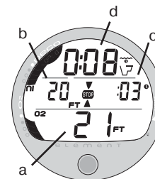
Рис. 36 Декомпрессионная остановка. Основной экран
