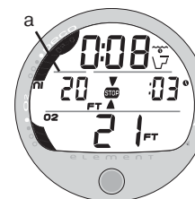
Рис. 4. Глубина декомпрессионной остановки
