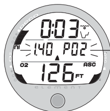
Рис. 48. Сигнал о достижении порогового значения парциального давления кислорода (установлено 1.4)
