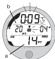
Рис. 37 Режим условного нарушения
