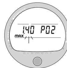
Рис. 22. Сигнальный индикатор парциального давления кислорода.
