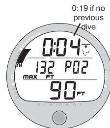
Рис. 54 Планировщик (данные скорректированы с учетом предыдущего погружения)
